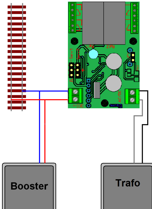
Tekening 2: DSDR aangesloten met aparte voeding.
