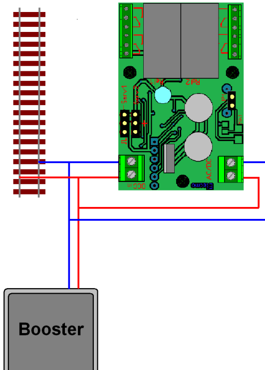
Tekening 1: Uitvoering DSDR: Aansluitschema met een gescheiden aansluiting voor het digitale signaal en voeding.
