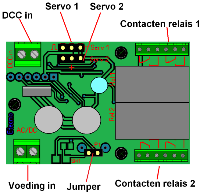
Overzicht van de aansluitingen van de servo decoder.
